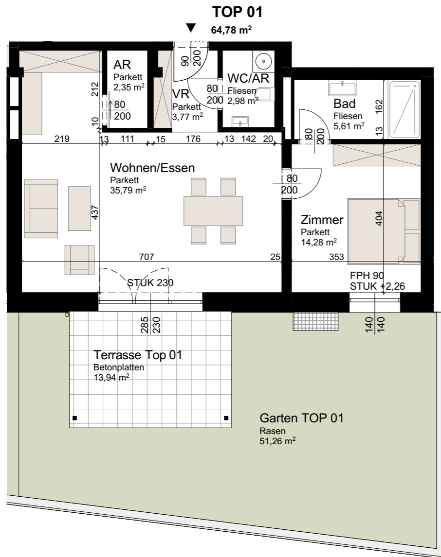
GRUNDRISS EG M 1:100
